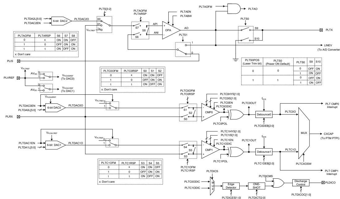
电源线收发器方框图
