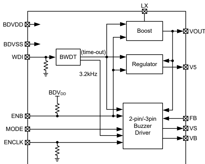
蜂鸣器驱动器方框图
