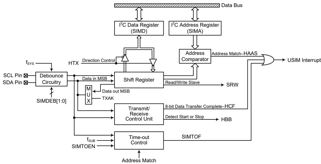
I²C 方框图
