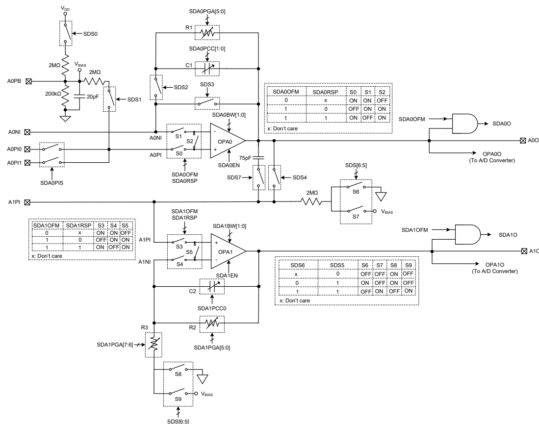
感烟探测器 AFE 方框图
