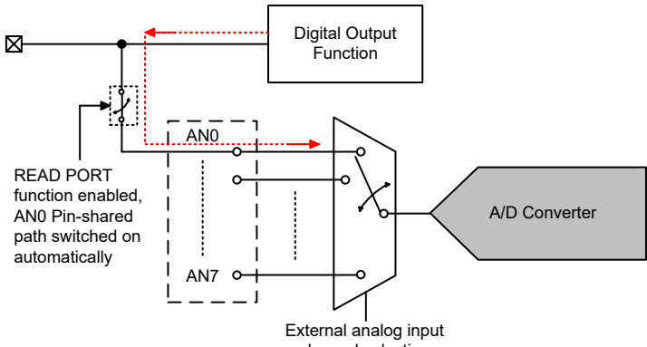
A/D 通道输入路径内部连接
