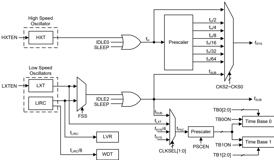
单片机时钟配置
