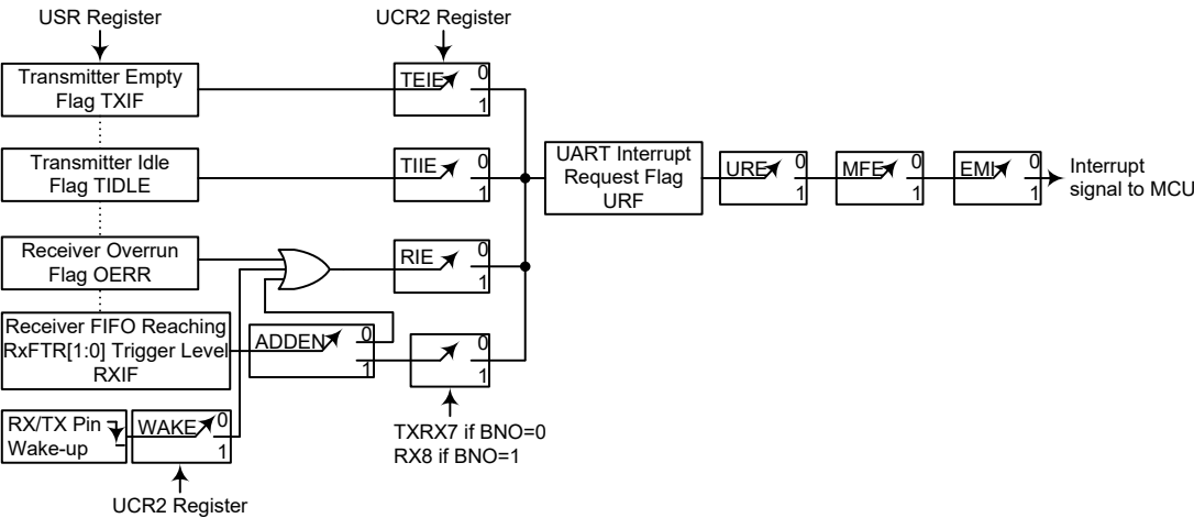
UART 中断框图
