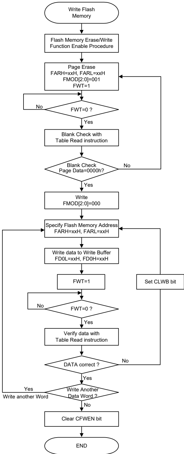
Flash 存储器非连续地址写入程序
