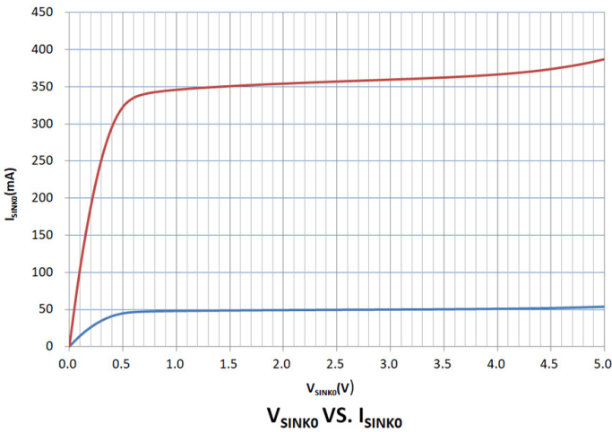
I_{SINK0} 电气特性曲线图
