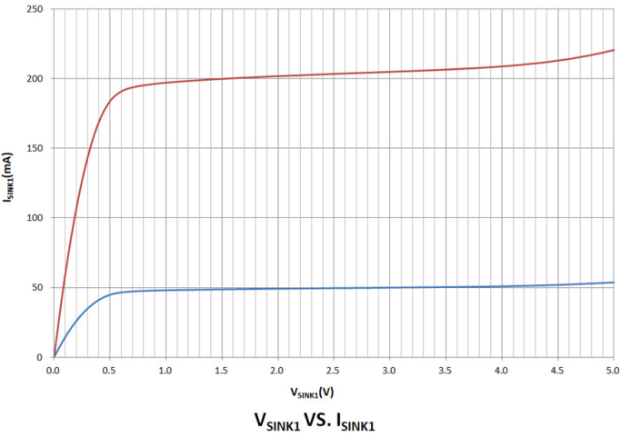
I_{SINK1} 电气特性曲线图
