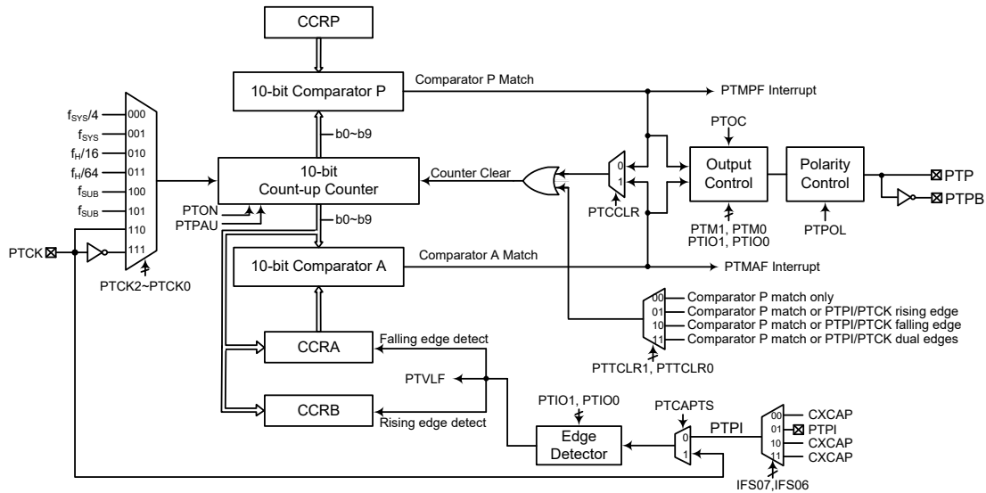
周期型 TM 方框图
