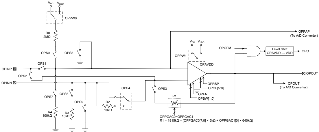
一氧化碳 / 燃气探测器 AFE 方框图
