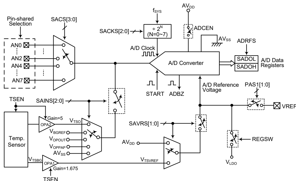
帶溫度传感器的 A/D 轉換器結構
