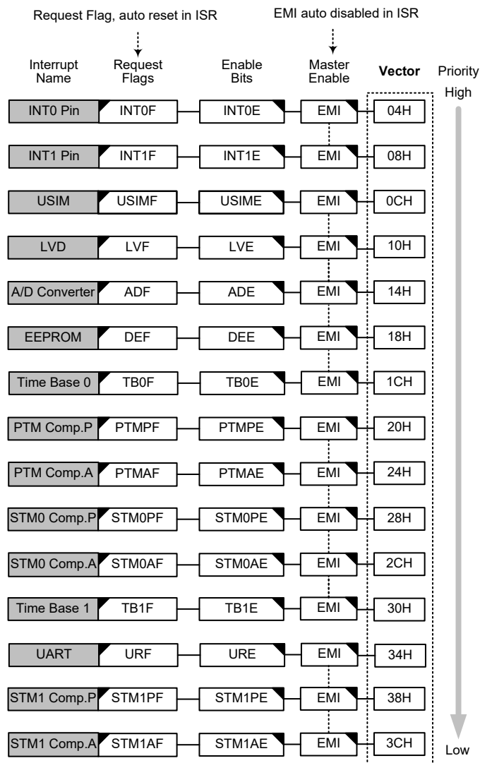
中断结构
