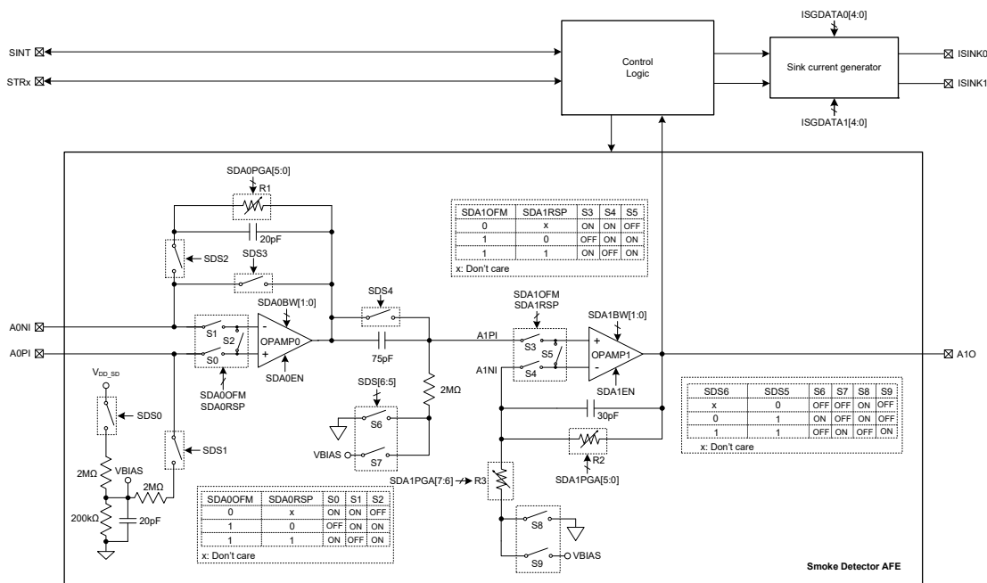
感烟探测器方框图
