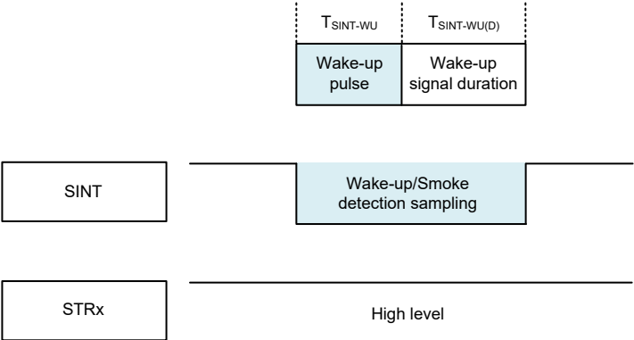
感烟探测唤醒
