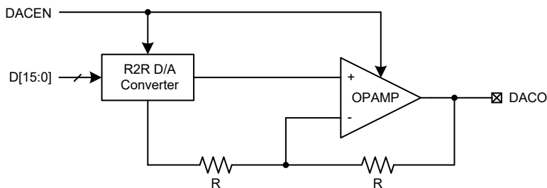
16-bit 语音 D/A 转换器结构
