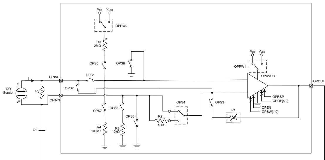
一氧化碳 / 燃气探测器 AFE 应用原理图
