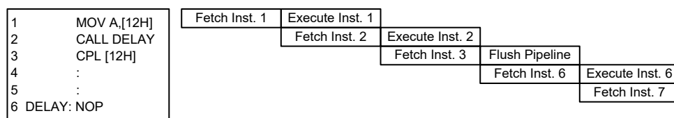
指令捕捉
