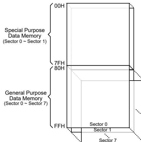
数据存储器结构
