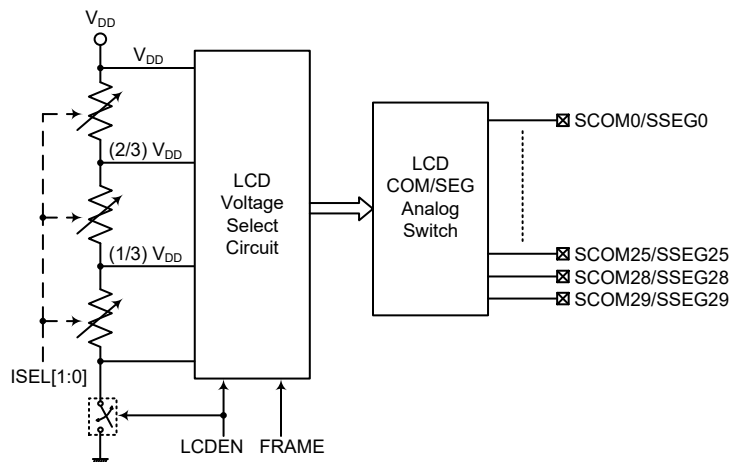
软件控制 LCD 驱动器结构
