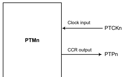
PTM 功能引脚方框图 (n=0~1)
