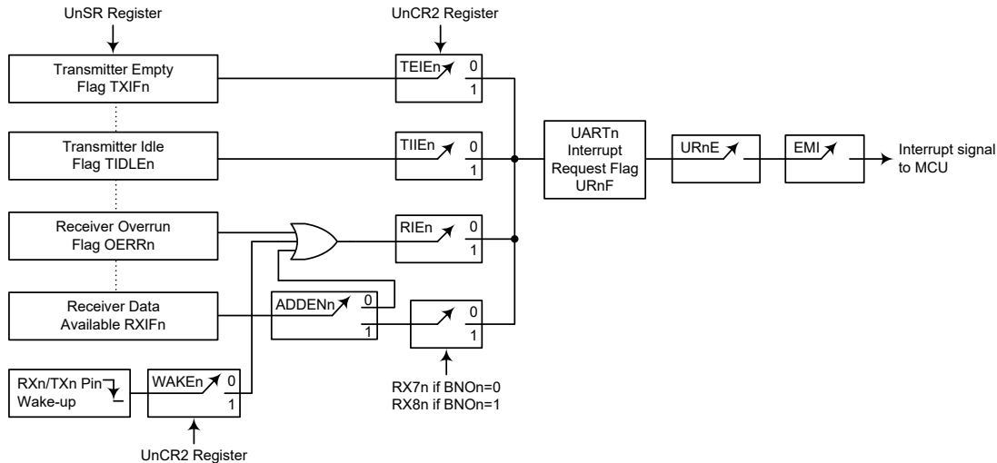
UART 中断框图 (n=0~1)
