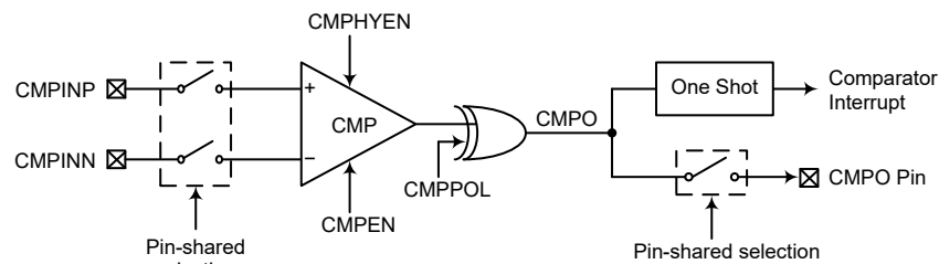
比较器
