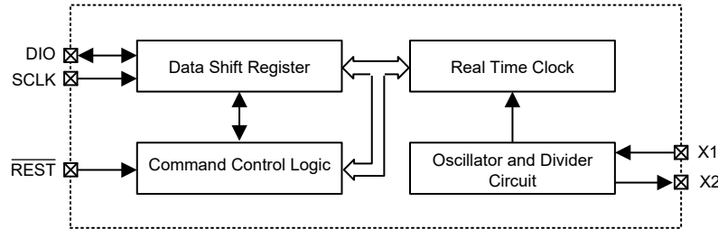
万年历方框图
