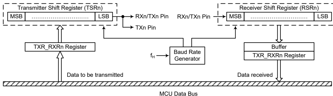
UARTn 数据传输方框图 - SWMn=1 (n=0~1)
