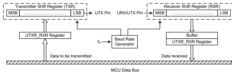
UART 数据传输方框图 – USWM=0
