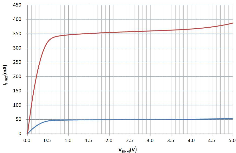
V_{SINK0} VS. I_{SINK0} I_{SINK0} 电气特性曲线图
