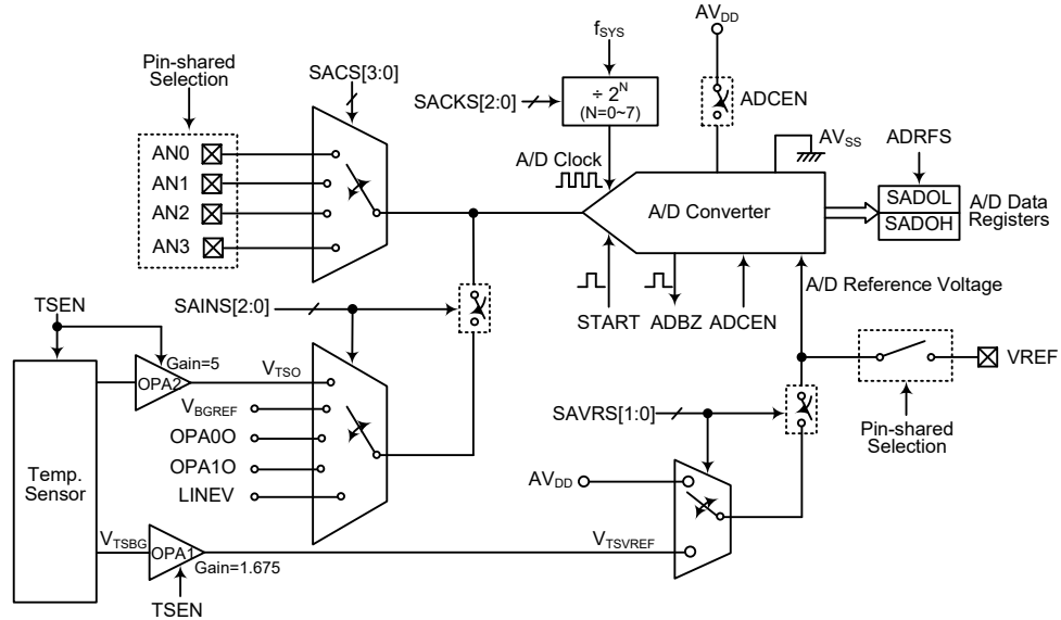
带温度传感器的 A/D 转换器结构
