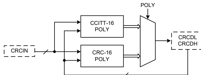
CRC 方框图
