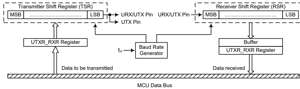
UART 数据传输方框图 - USWM=1
