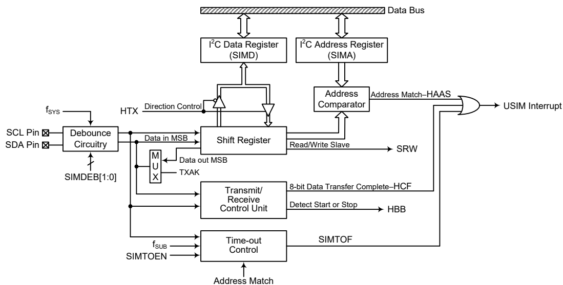
I²C 方框图
