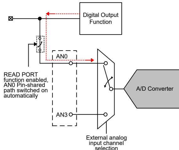
A/D 通道输入路径内部连接
