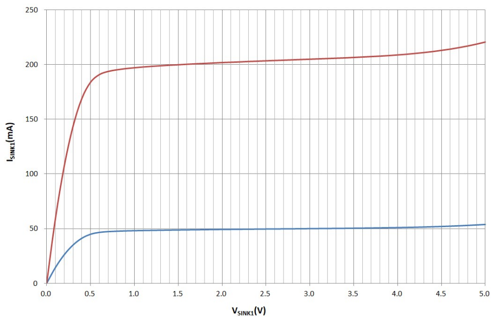
V_{SINK1} VS. I_{SINK1} I_{SINK1} 电气特性曲线图
