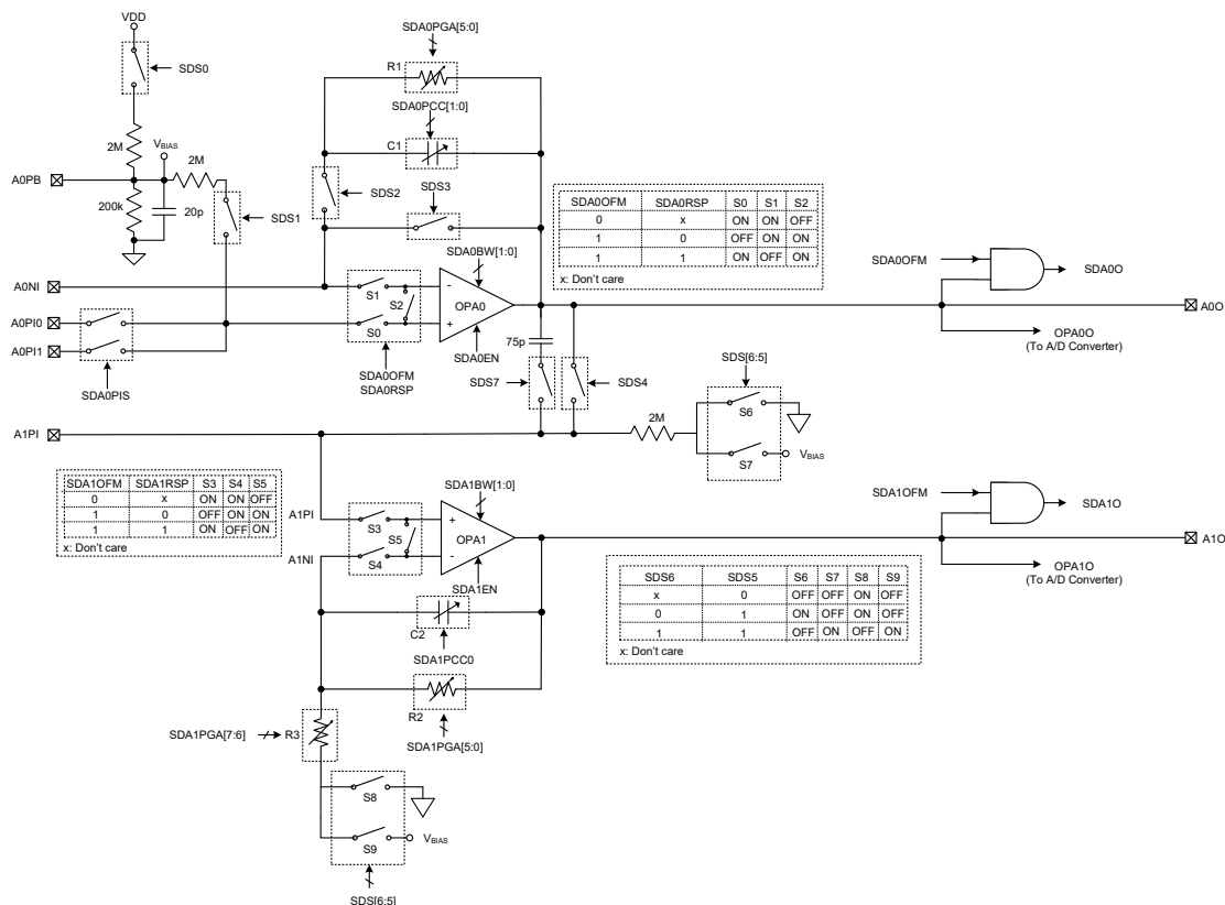
感烟探测器 AFE 方框图
