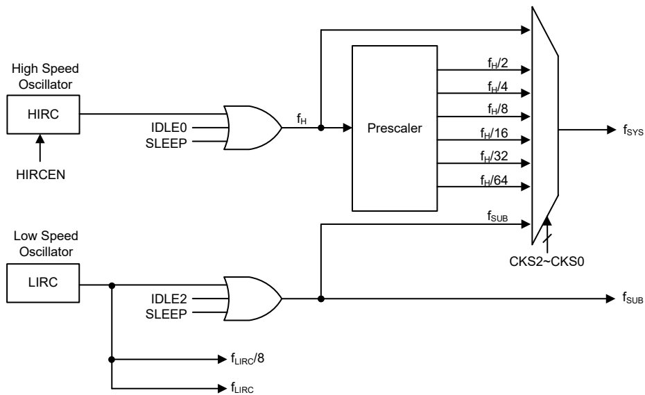
系统时钟配置
