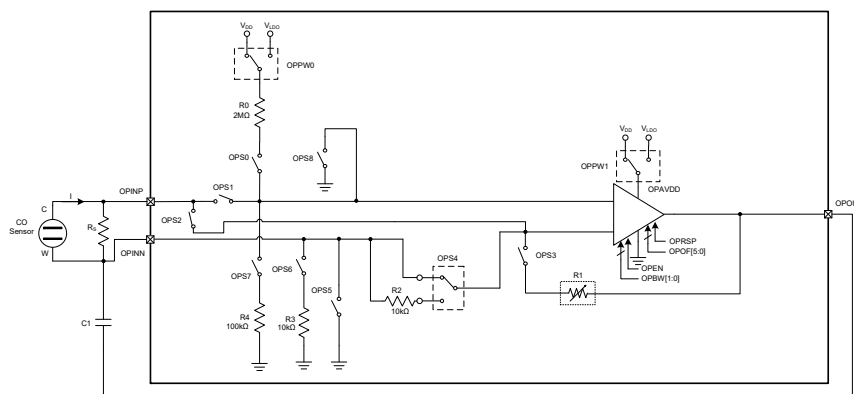
CO / 燃气探测器 AFE 应用原理图
