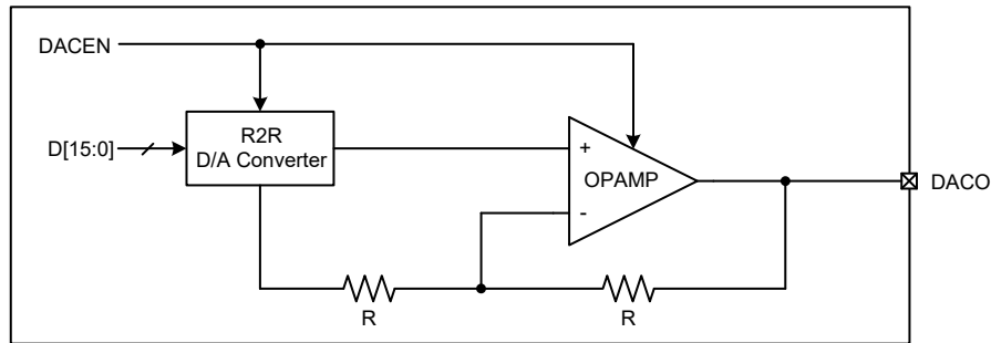
16-bit 语音 D/A 转换器结构
