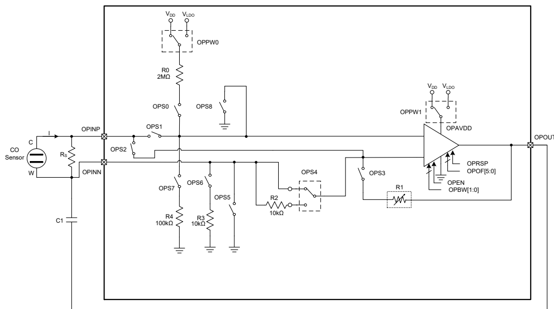
CO / 燃气探测器 AFE 应用原理图
