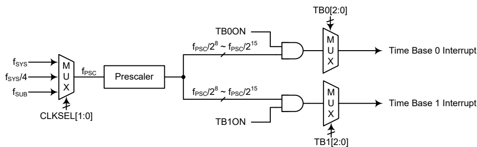
时基中断
