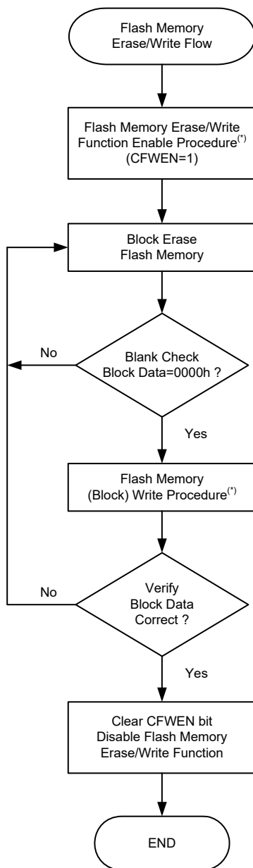
Flash 存储器擦 / 写流程图
