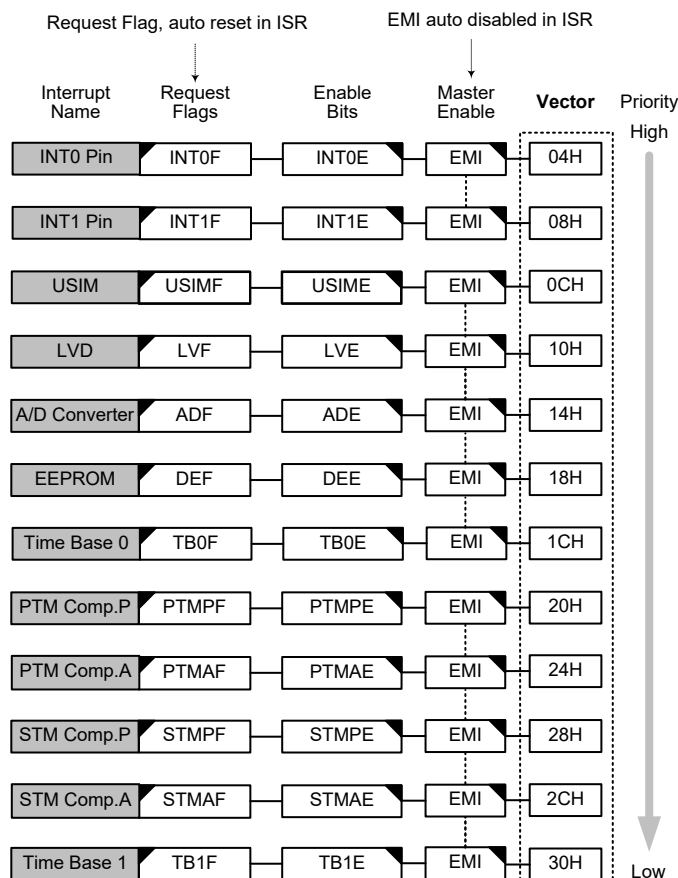
中断结构
