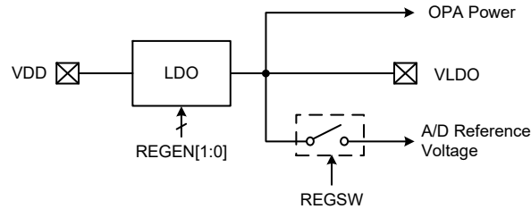
LDO 方框图
