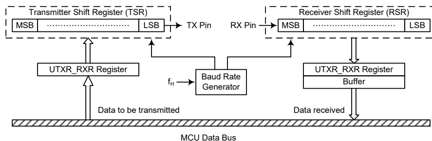
UART 数据传输方框图
