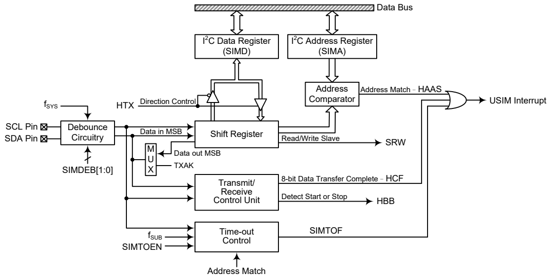
I²C 方框图
