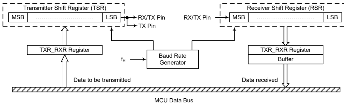
UART 数据传输方框图 – SWM=1
