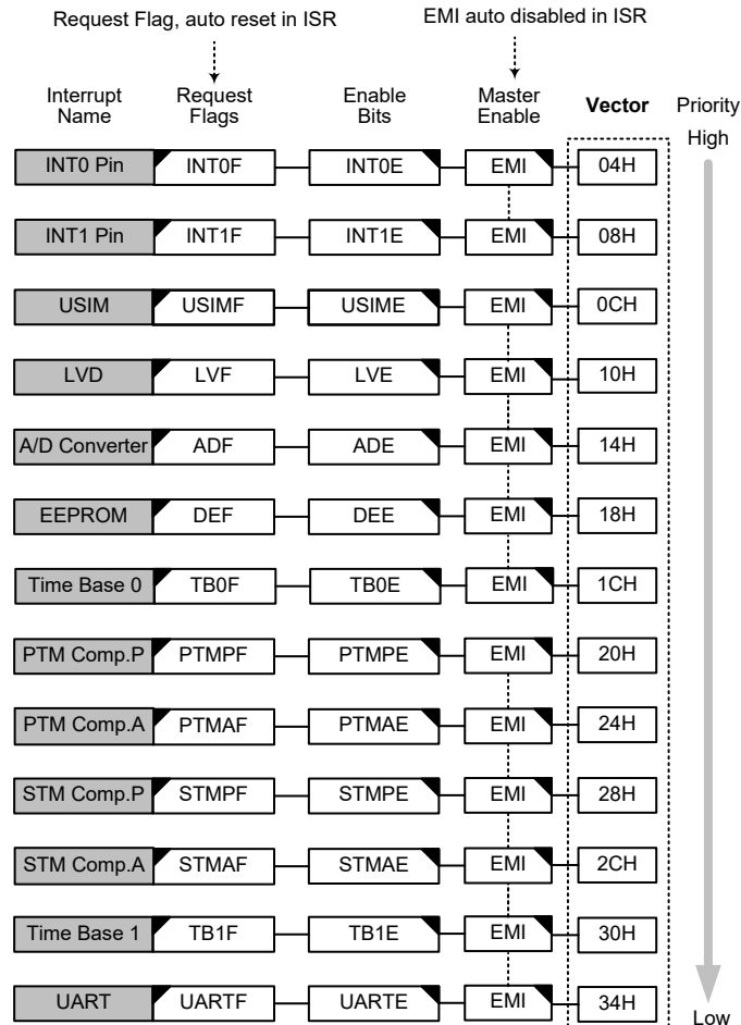
中断结构
