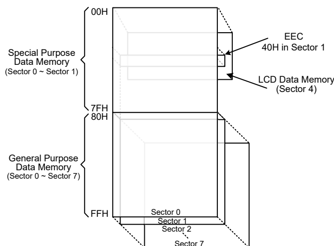
数据存储结构
