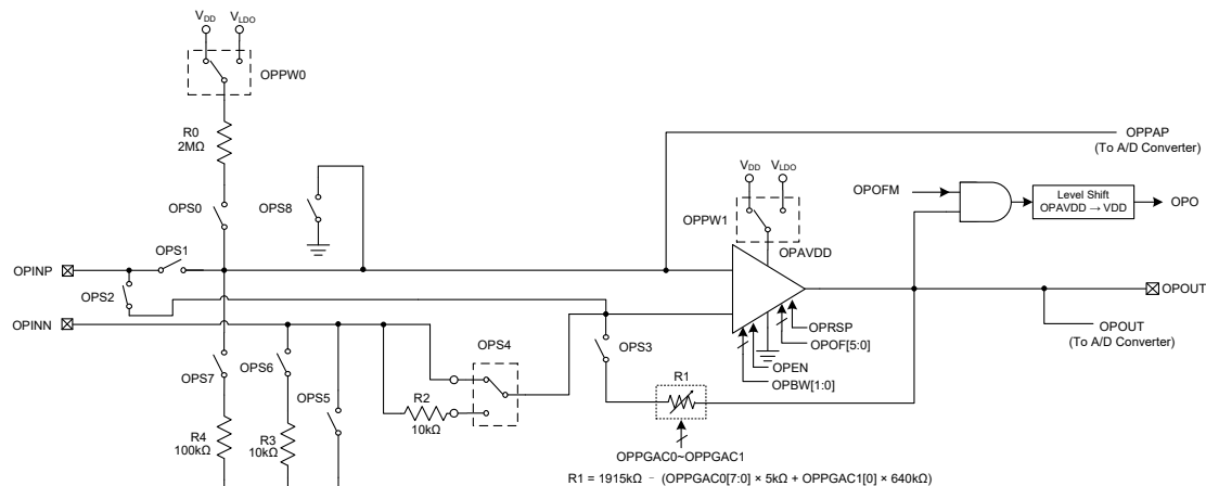
CO / 燃气探测器 AFE 方框图
