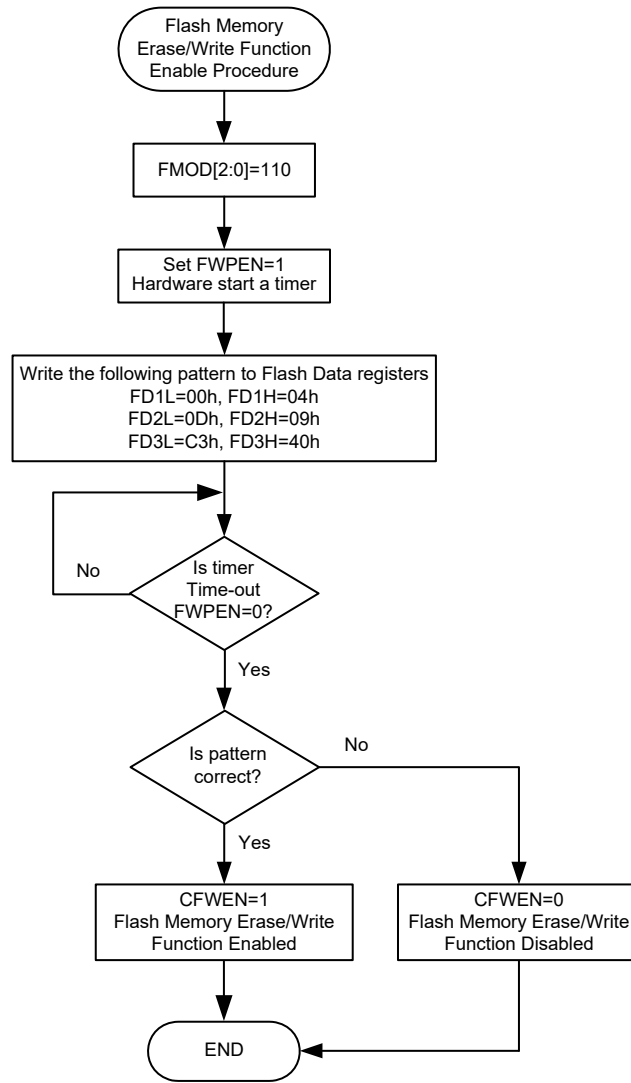
Flash 存储器擦 / 写使能程序
