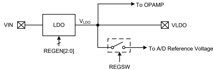
LDO 稳压器方框图
