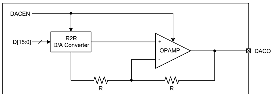
16-bit 语音 D/A 转换器结构
