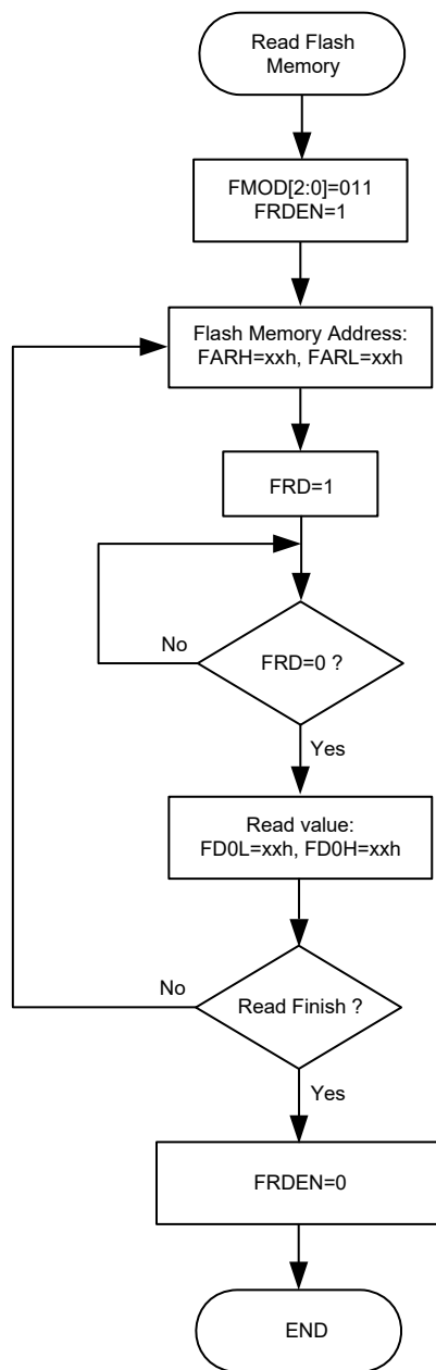
Flash 存储器读出程序
