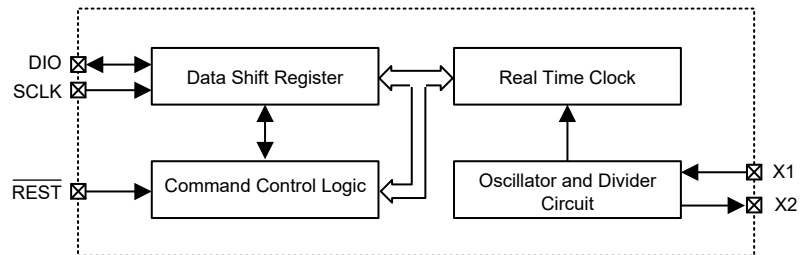
万年历方框图
