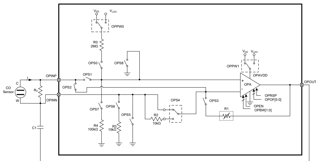
CO / 燃气探测器 AFE 应用原理图
