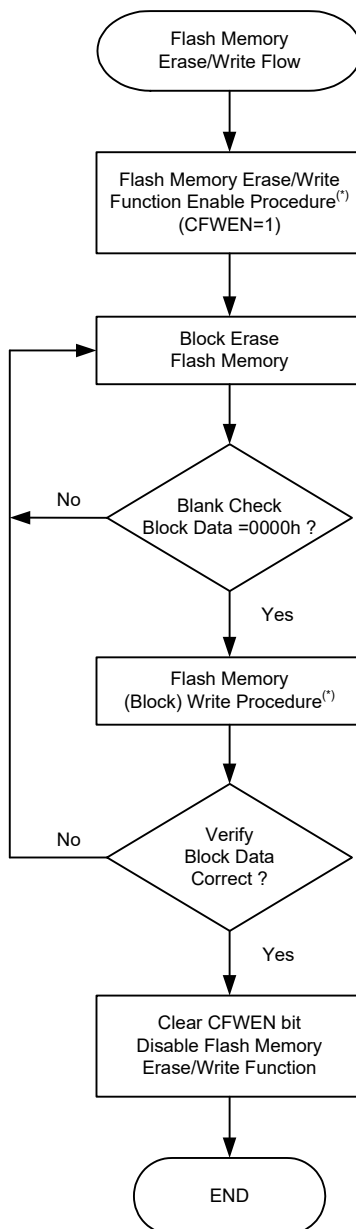
Flash 存储器擦 / 写流程图
