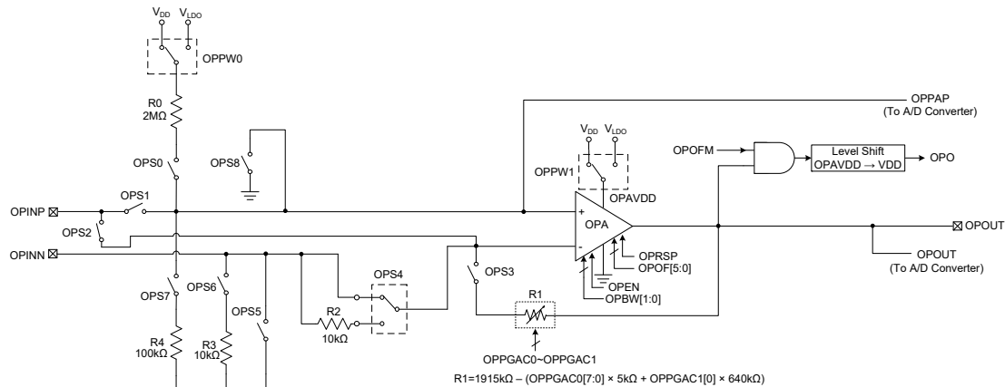
CO / 燃气探测器 AFE 方框图
