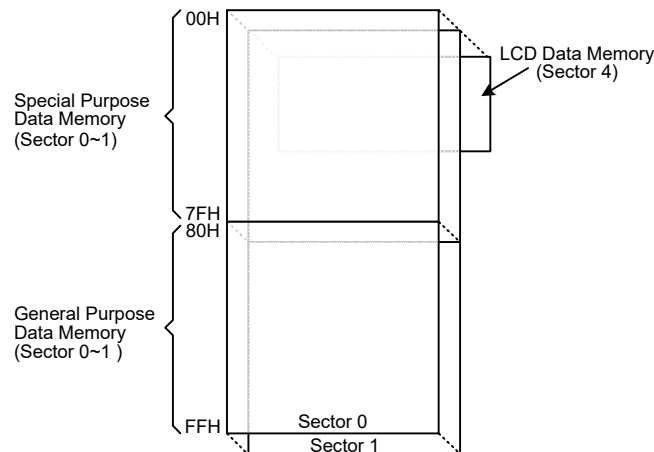
数据存储器结构
