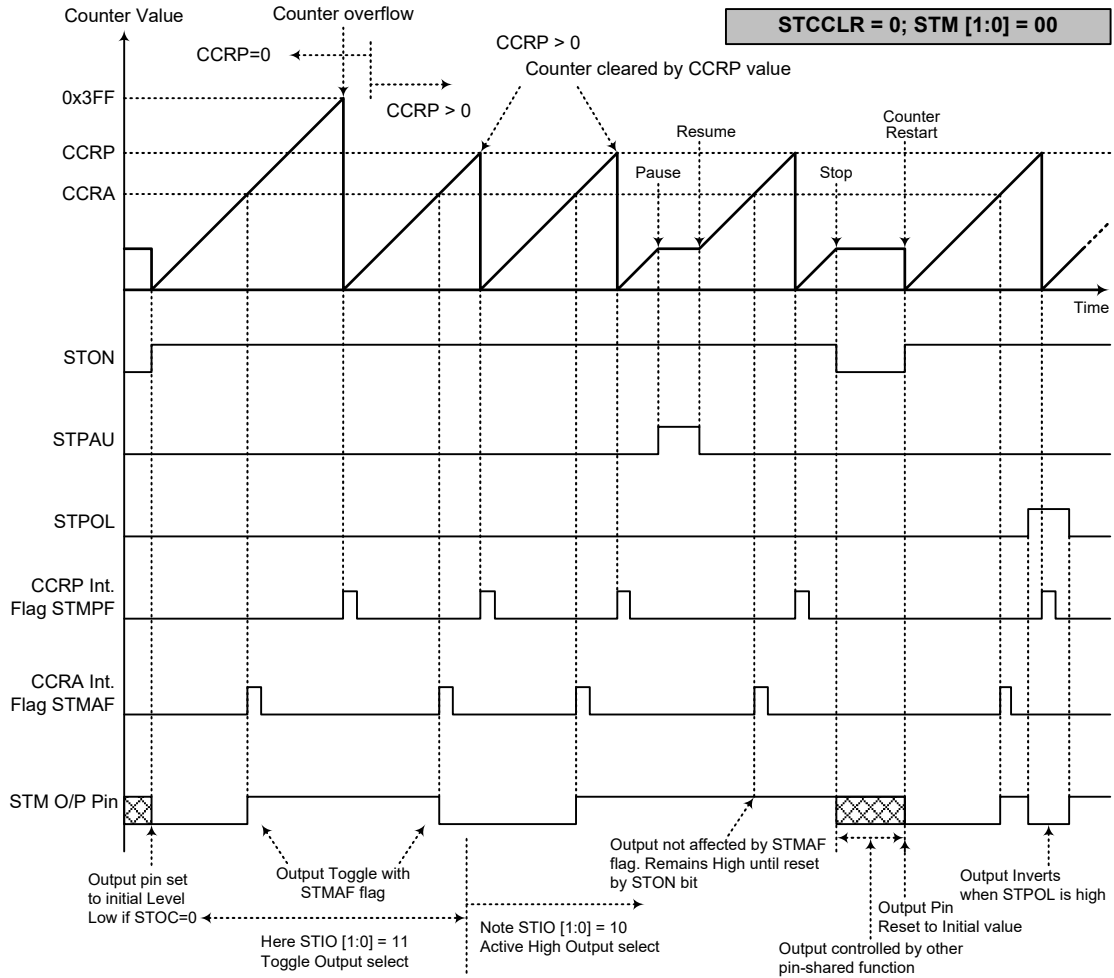
比较匹配输出模式 – STCCLR=0
