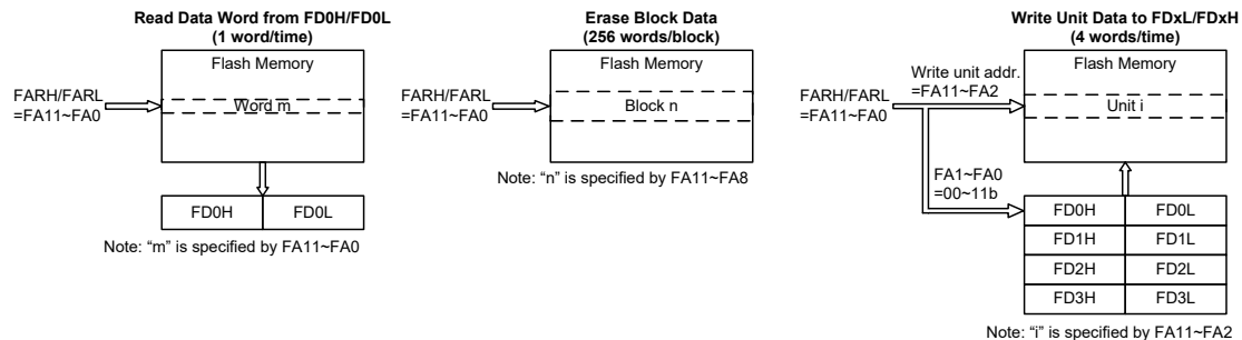
Flash 存储器 IAP 读 / 擦 / 写结构
