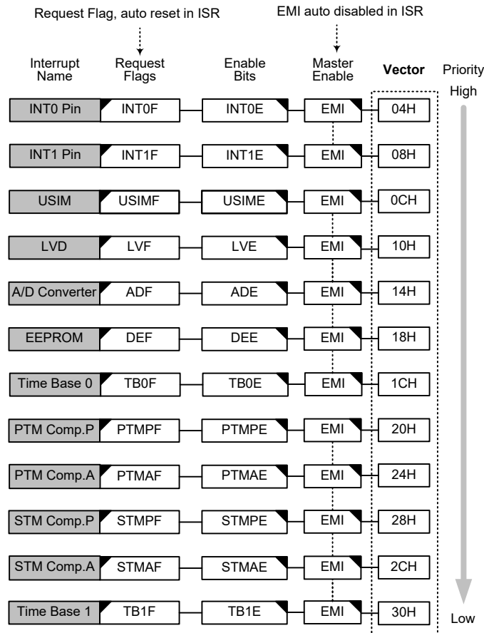
中断结构
