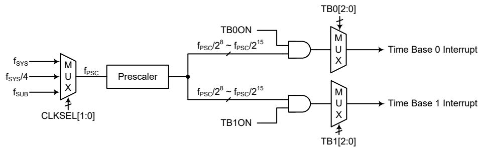
时基中断
