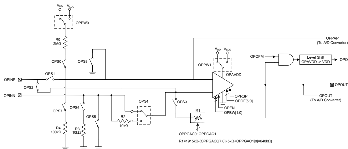
CO / 燃气探测器 AFE 方框图
