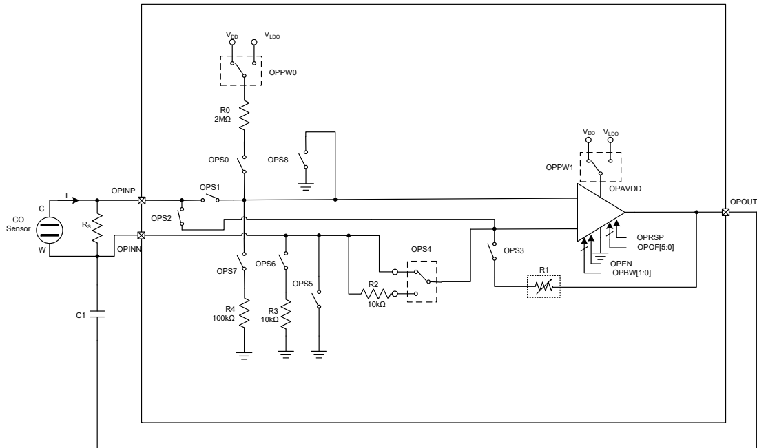
CO / 燃气探测器 AFE 应用原理图
