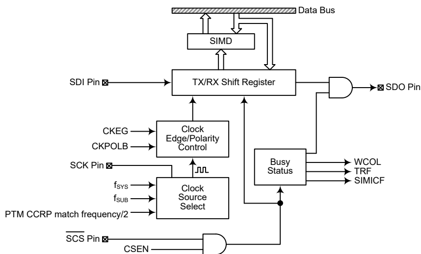
SPI 方框图
