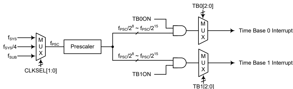
时基中断
