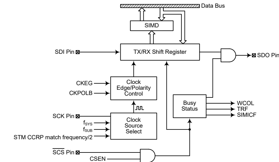
注：对于 BA45F5740-2 芯片，SCS 引脚未引出，SPI 功能不可用。 SPI 方框图
