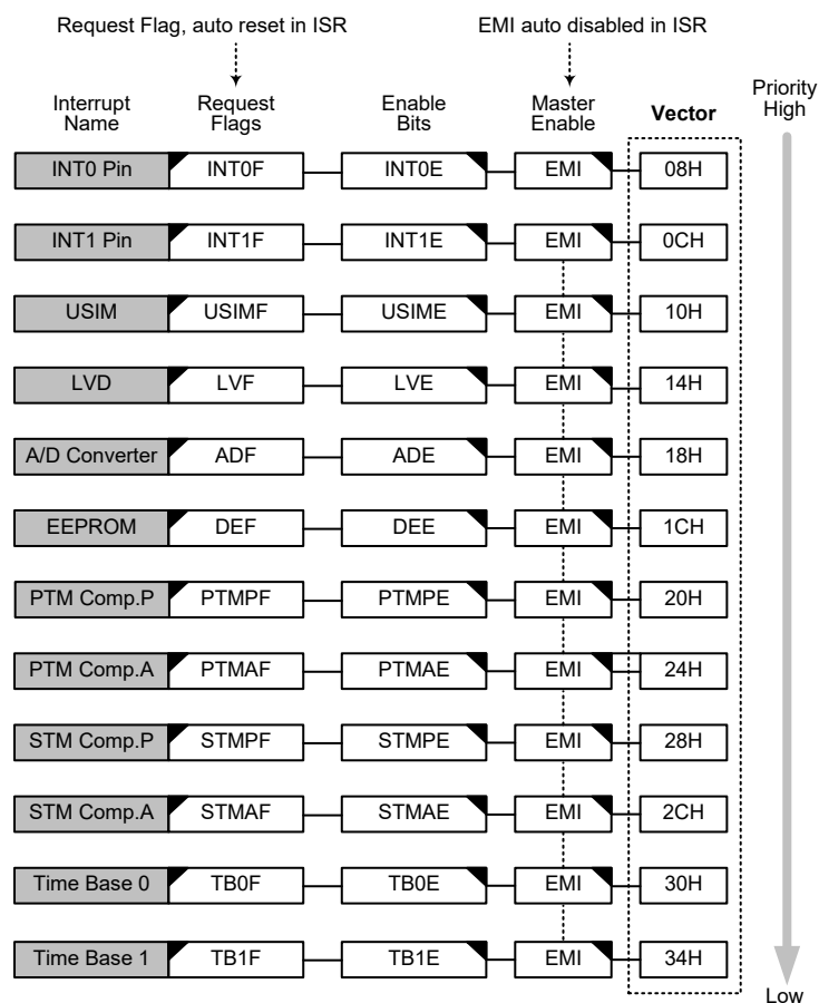
中断结构
