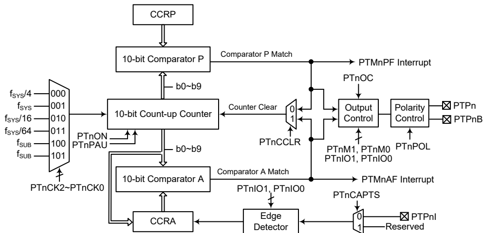
周期型 TM 方框图 ( n=0 )
