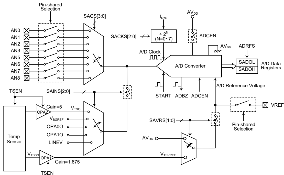
带温度传感器的 A/D 转换器结构图
