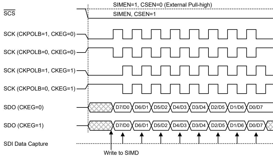
SCK 主机模式时序
