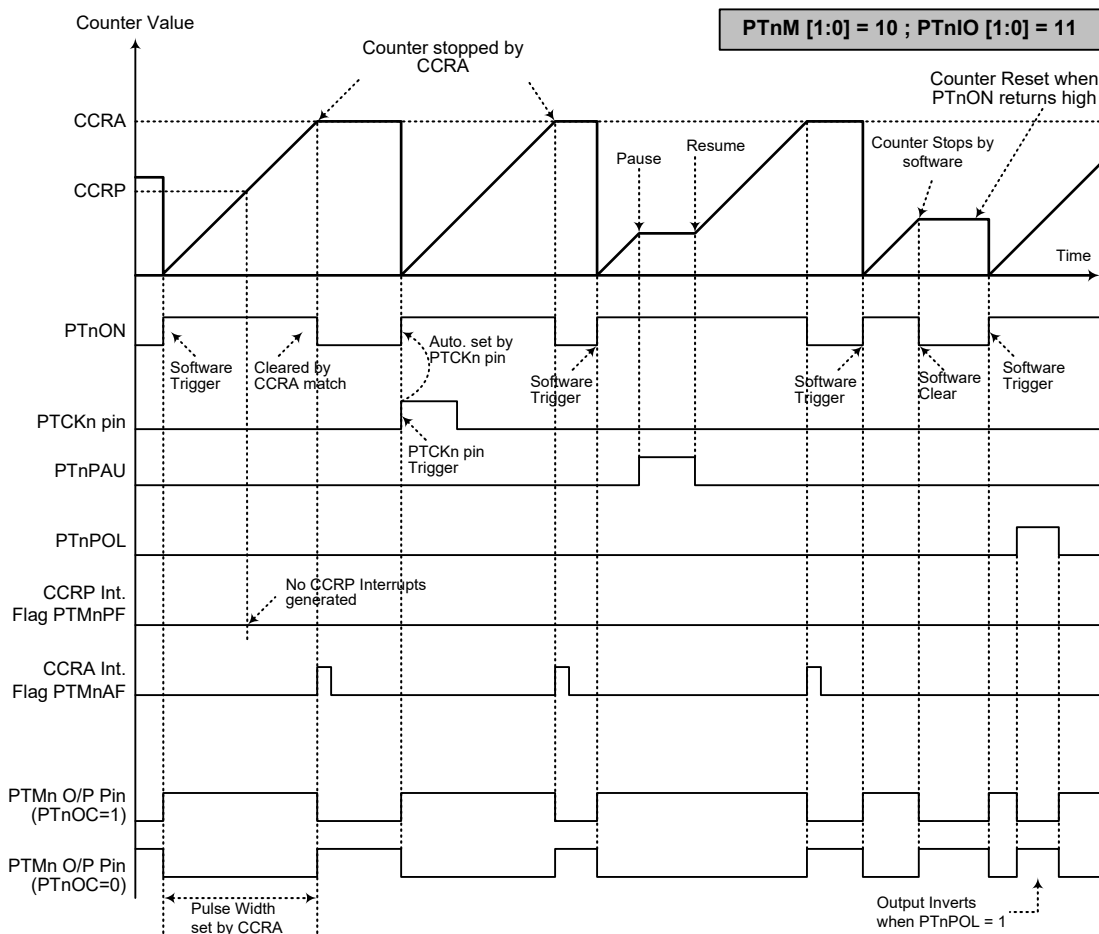
单脉冲输出冲模式 (n=0~1)
