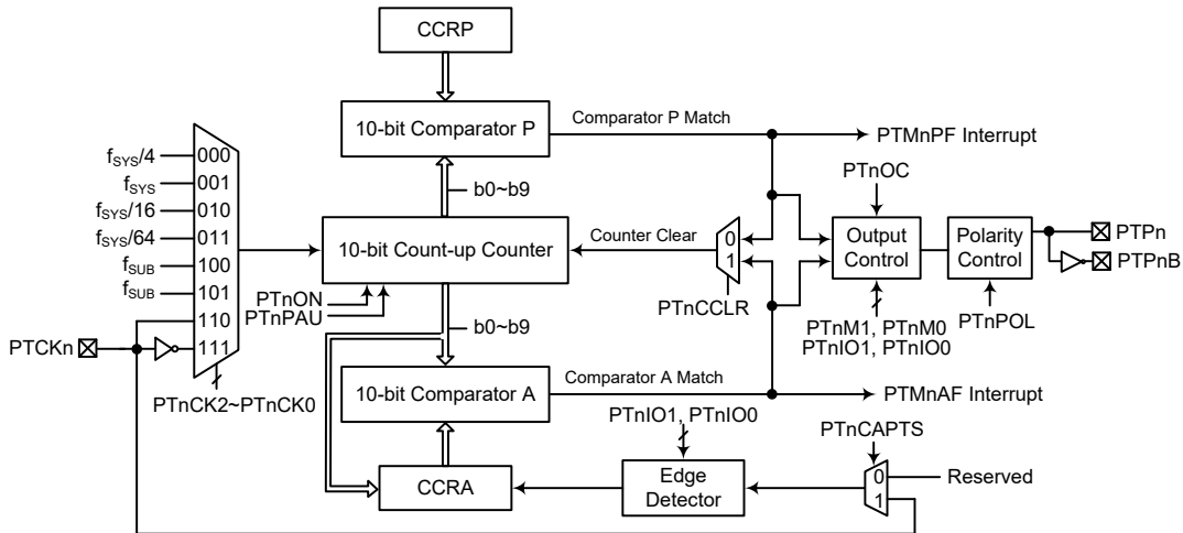
周期型 TM 方框图 (n=1)
