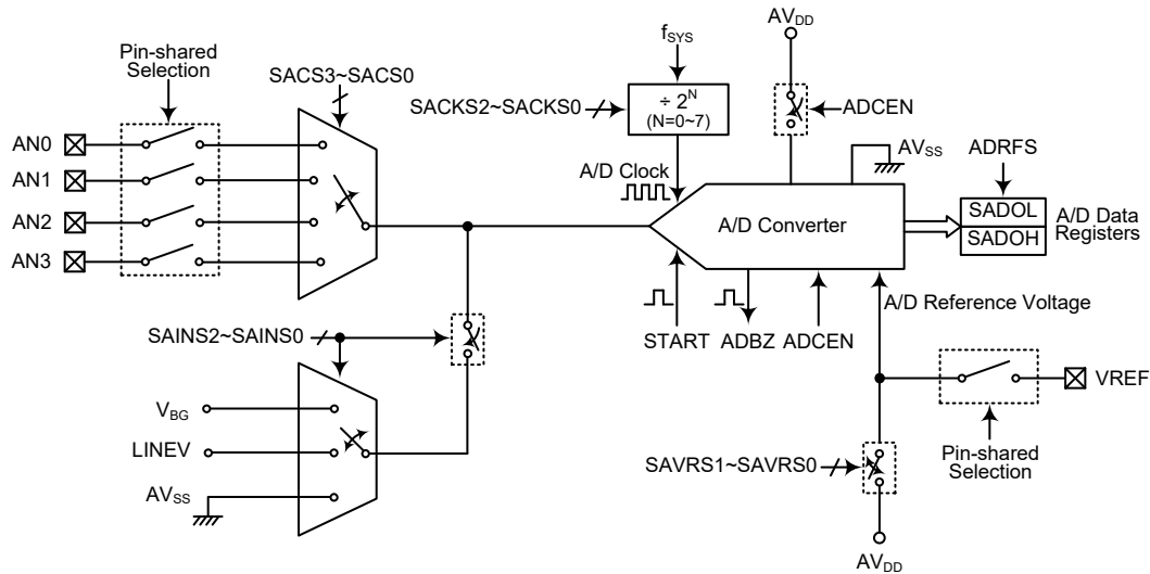
A/D 转换器结构
