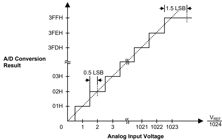
理想的 A/D 转换功能
