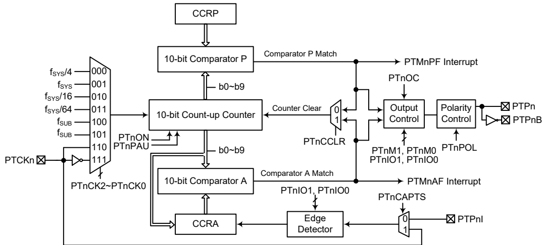
周期型 TM 方框图 (n=0)
