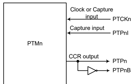
PTMn 功能引脚方框图 (n~1)
