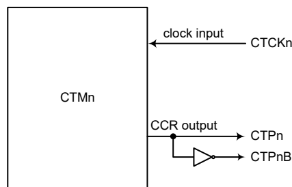
CTMn 功能引脚方框图 (n~1)
