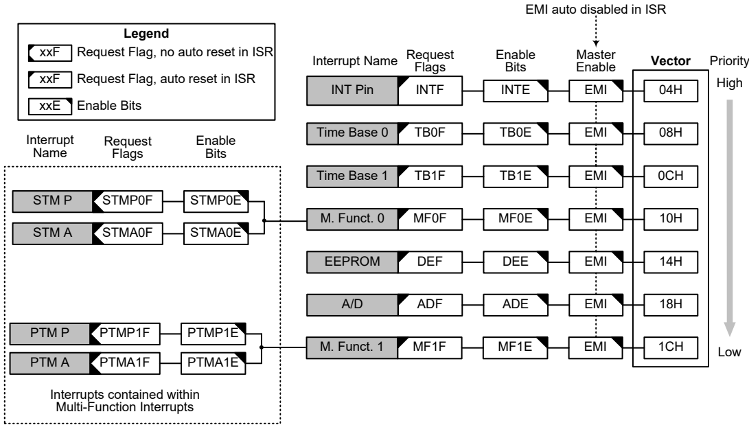
中断结构
