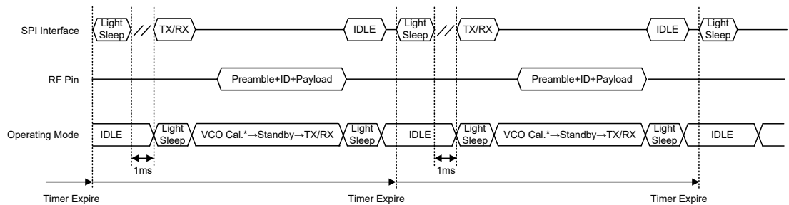
FIFO 模式 RX 时序图
