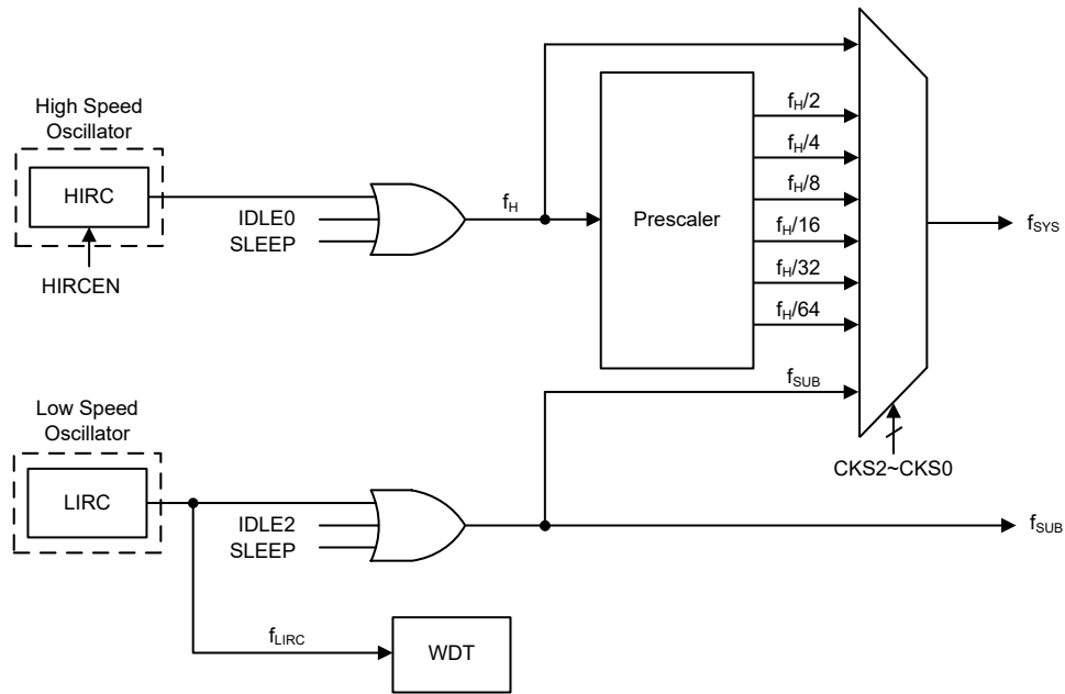
系统时钟配置
