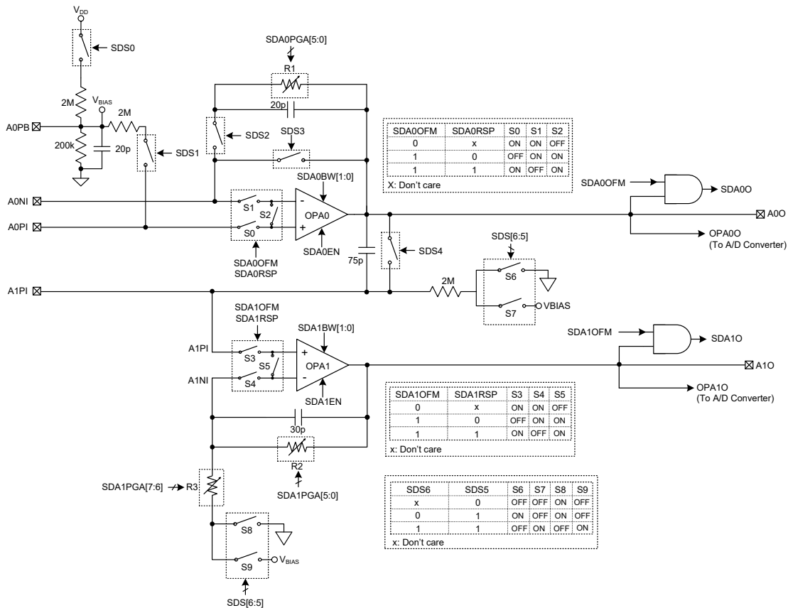
烟感器 AFE 方框图
