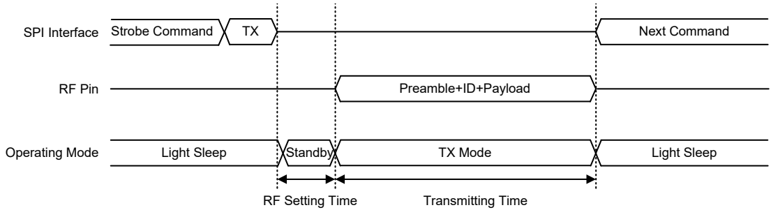
FIFO 模式 TX 时序图
