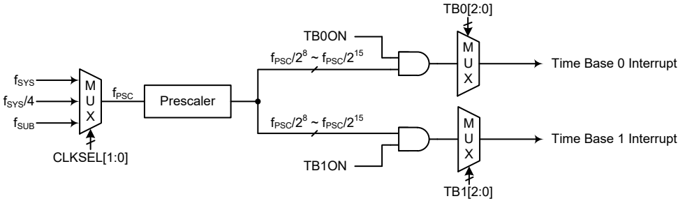
时基中断
