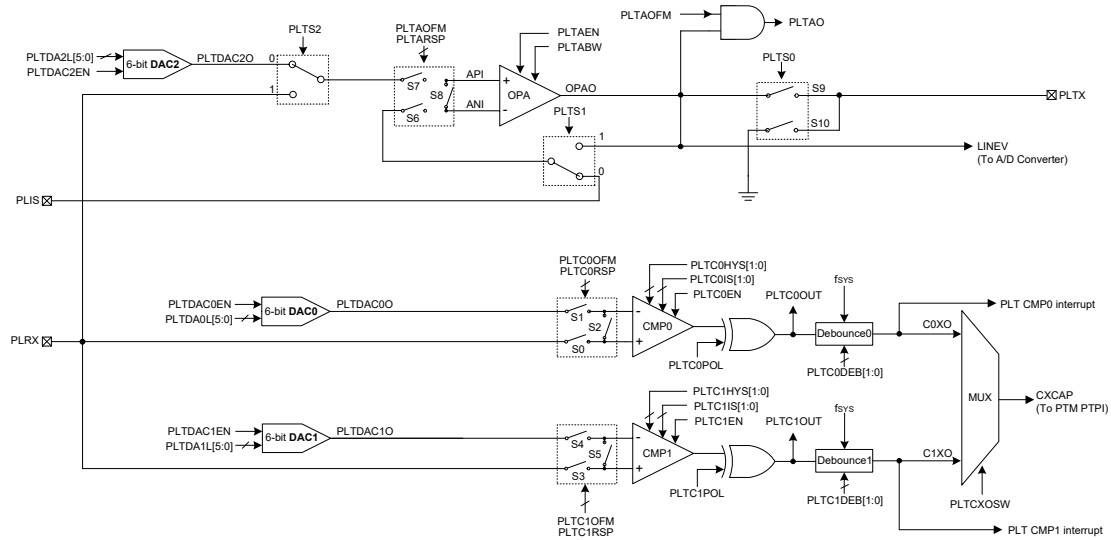
电源线数据收发器方框图
