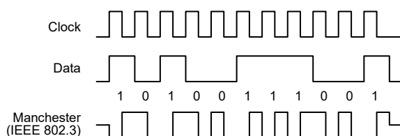
曼彻斯特码举例
