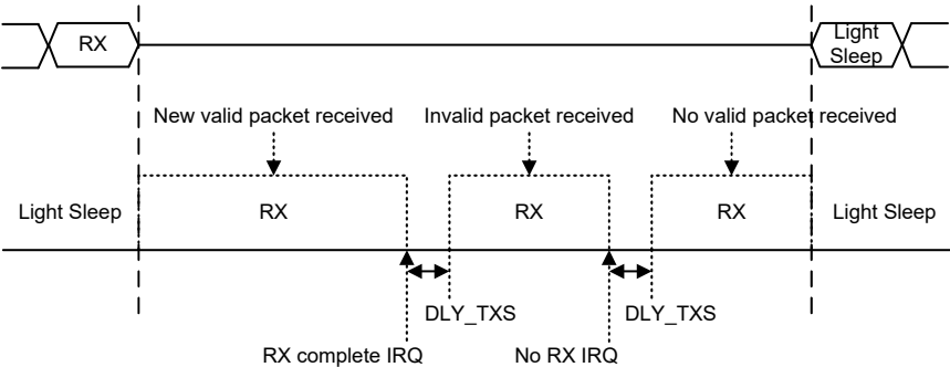
连续 RX 模式
