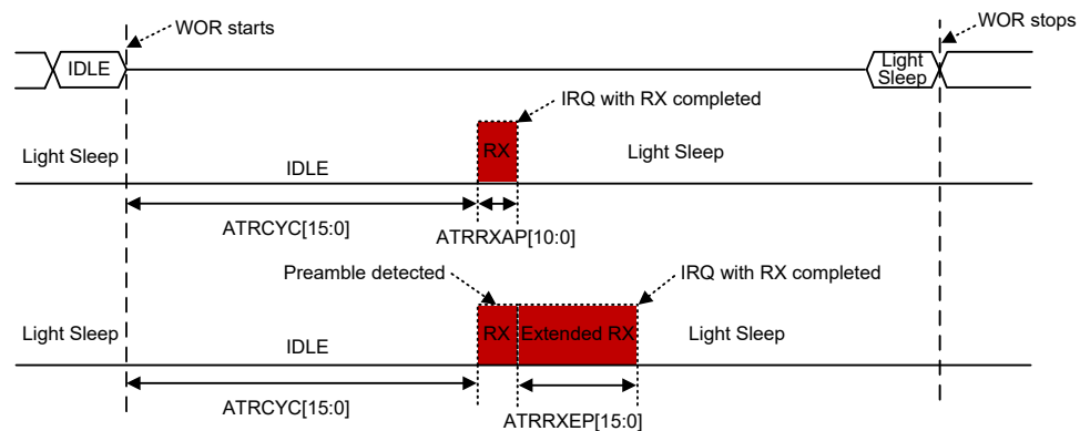
接收到传入数据后停止 WOR
