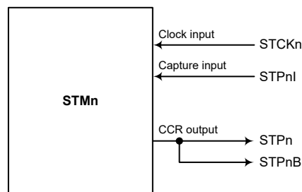
STMn 功能引脚方框图 (n~1)
