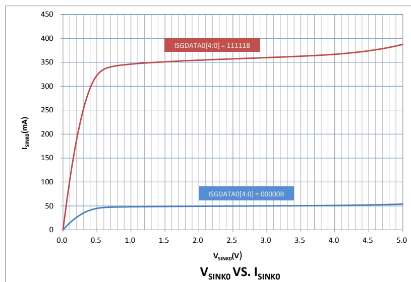
I_{SINK0} 特性曲线图
