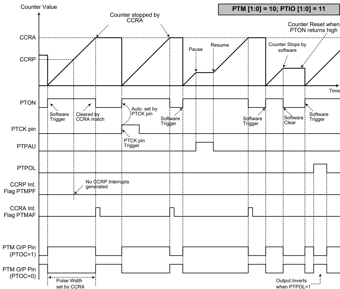
单脉输出冲模式
