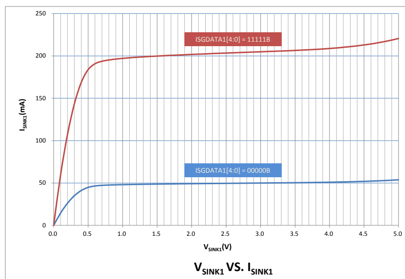
I_{SINK1} 特性曲线图
