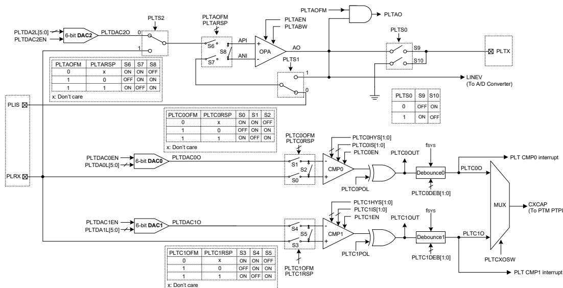
电源线数据收发器方框图
