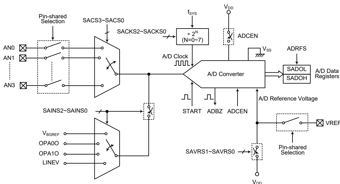
A/D 转换器结构
