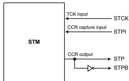
STM 功能方框图
