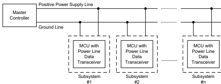
电源线数据收发器系统方框图
