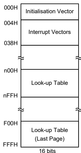
程序存储器结构
