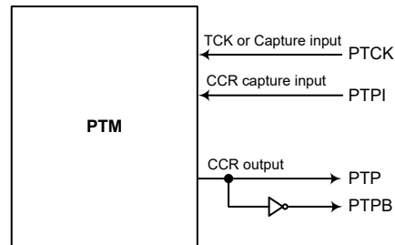
PTM 功能方框图
