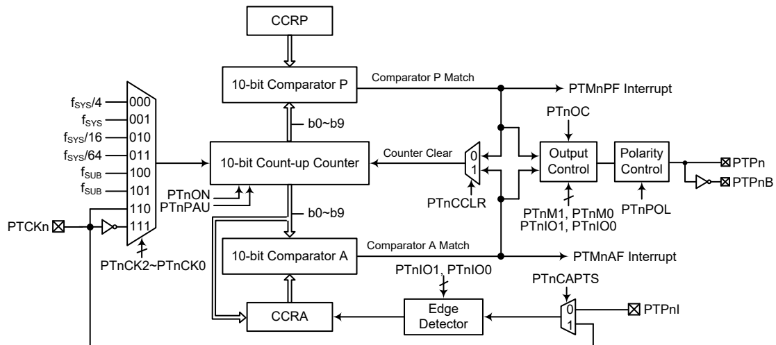
周期型 TM 方框图 (n=0)
