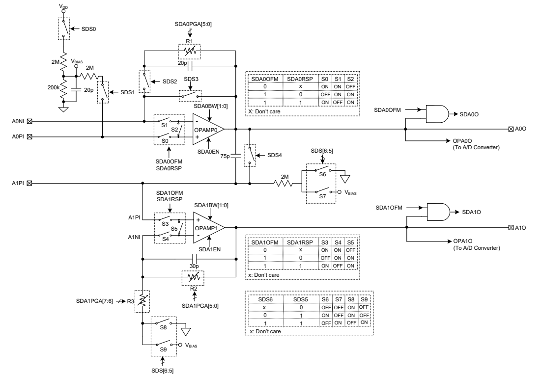
感烟探测器 AFE 方框图
