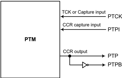
PTM 功能方框图
