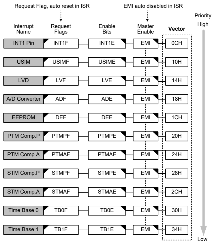
中断结构
