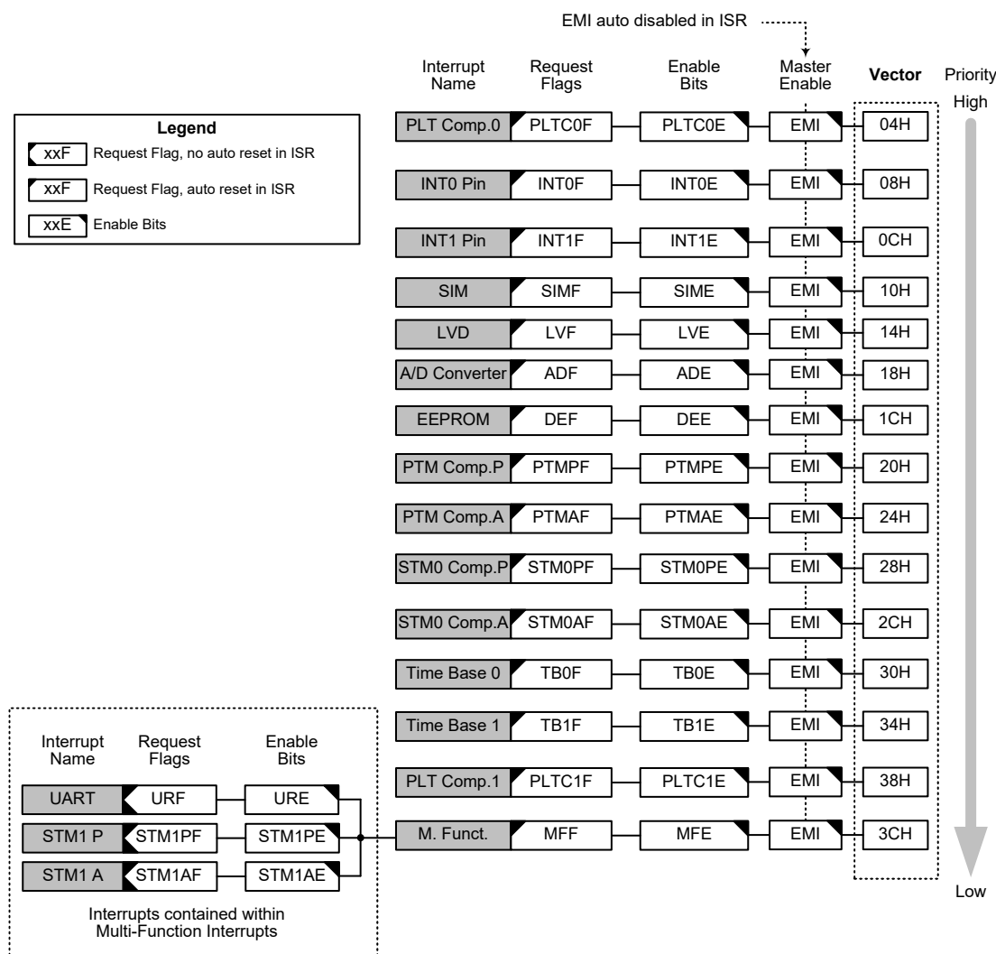
中断结构
