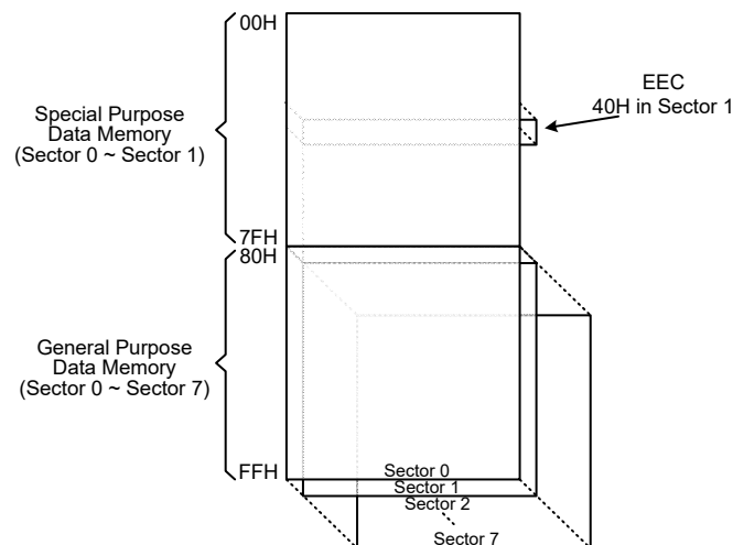
数据存储结构
