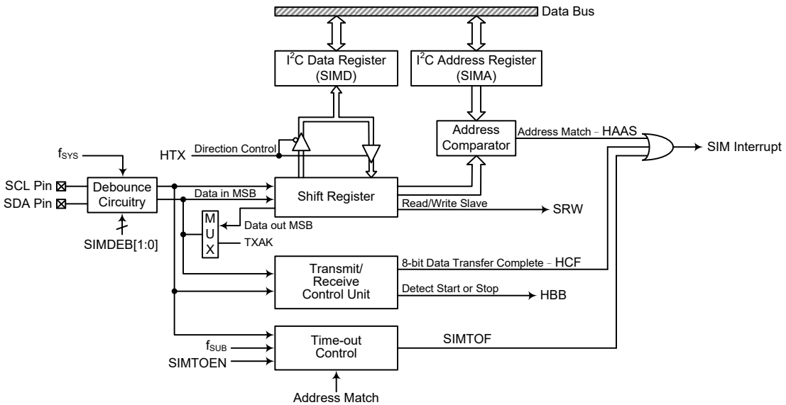
I²C 方框图
