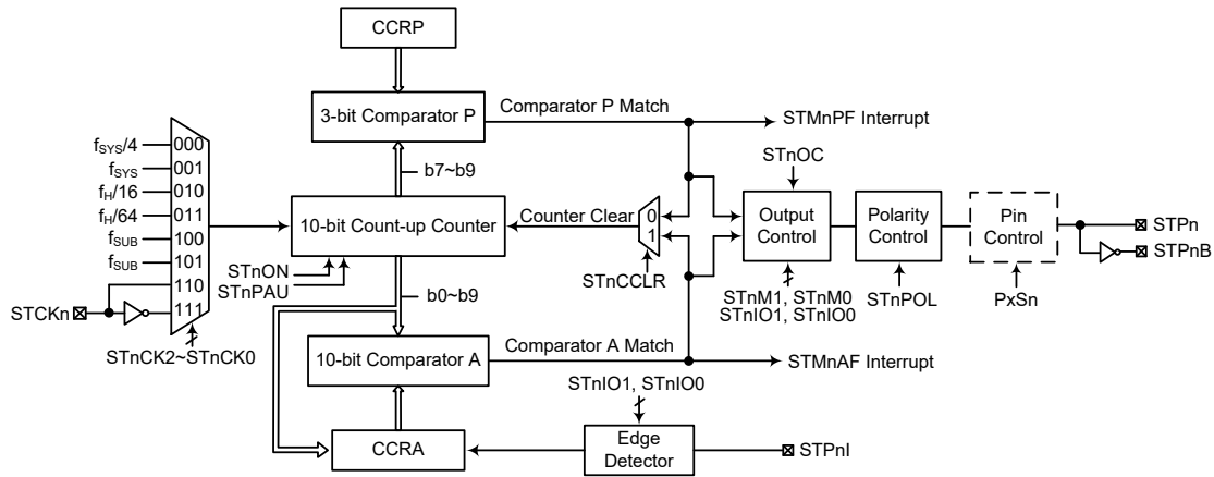
标准型 TM 方框图 (n=0~1)
