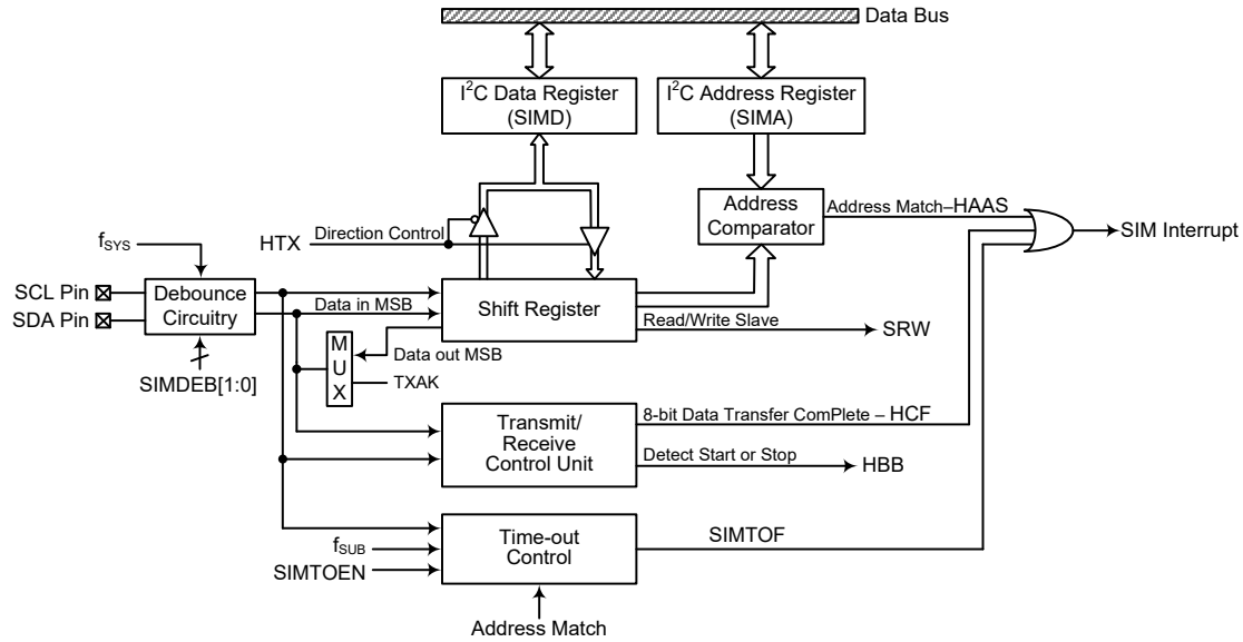
I²C 方框图
